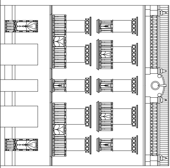
ALZADO OALLE
