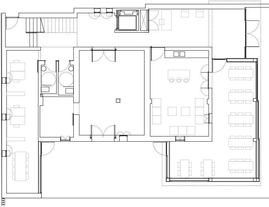
PLANTA BAJA
