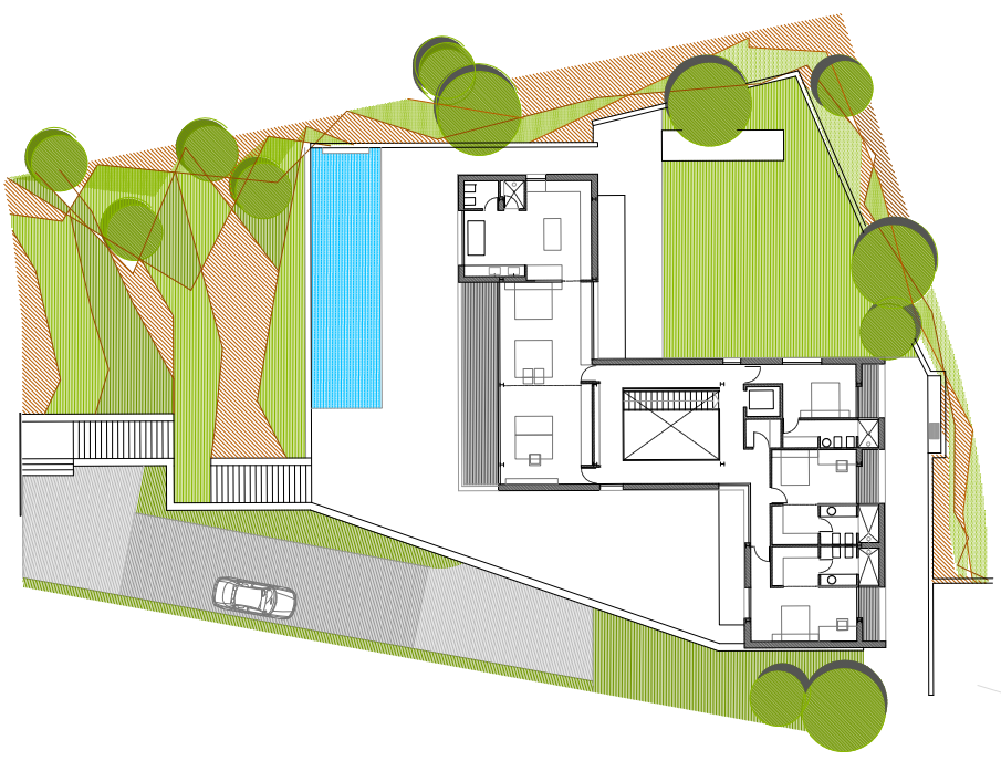
PLANTA PRIMERA
